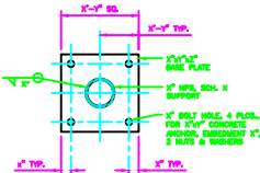
DET. 2 BASE PLATE w/PIPE
